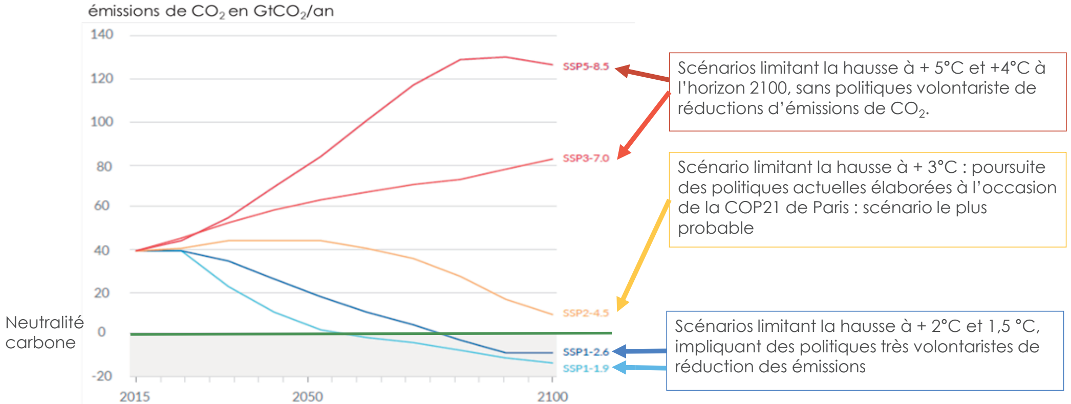
Émissions de CO 2 selon les scénarios étudiés par le GIEC Source : Giec, 1er groupe de travail, 2021
